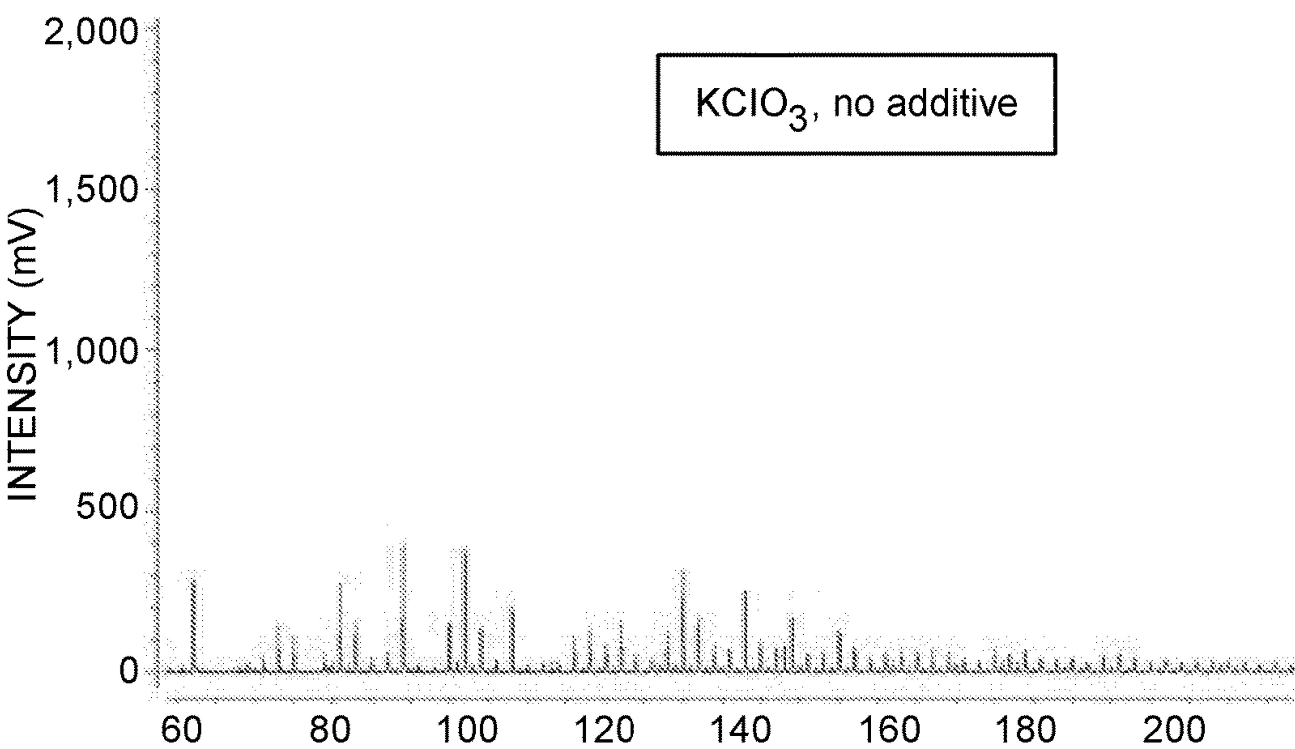
FIG. 10B
