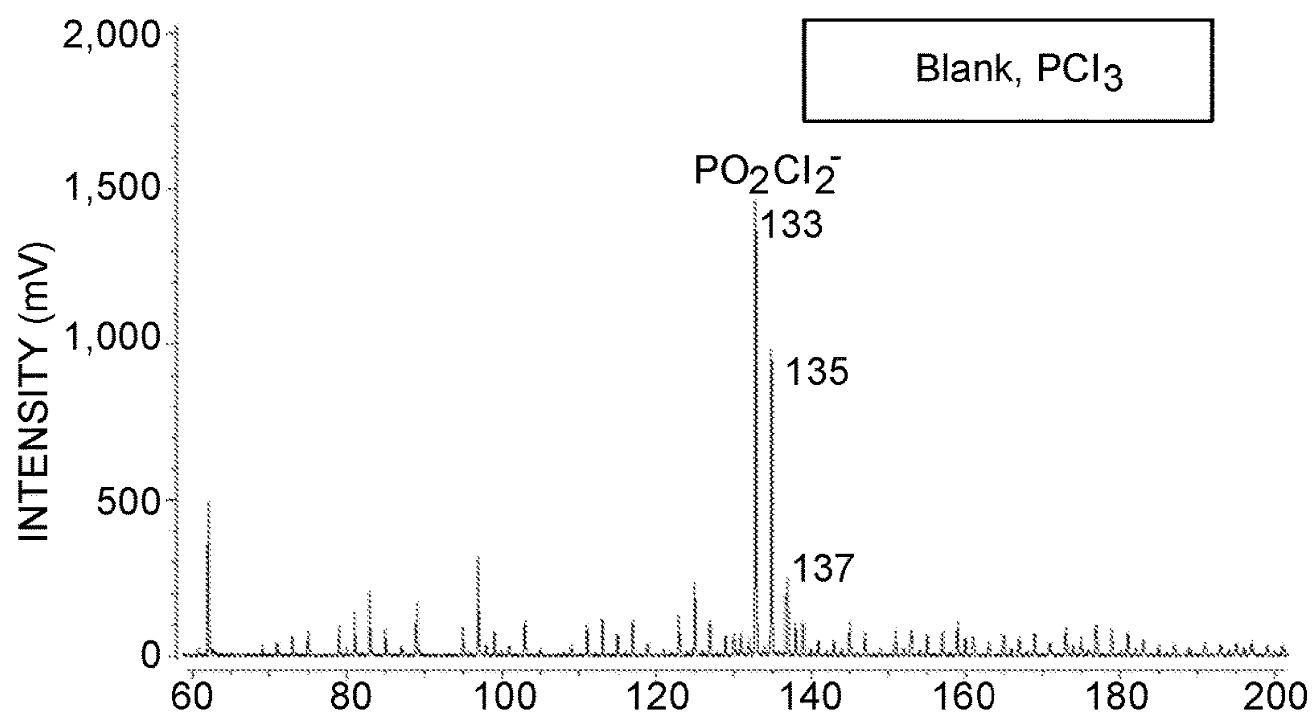
FIG. 11A
