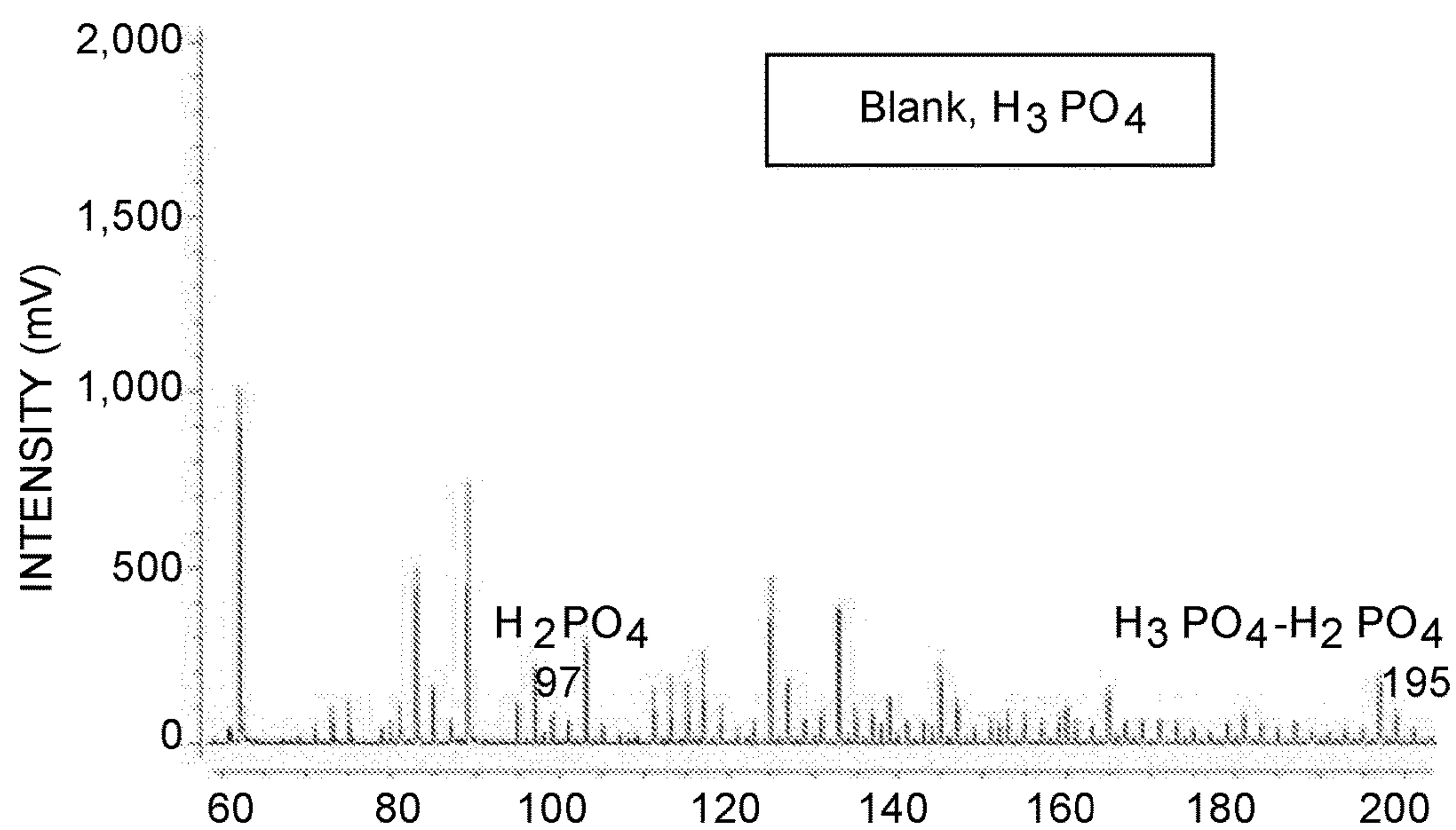
FIG. 10C
