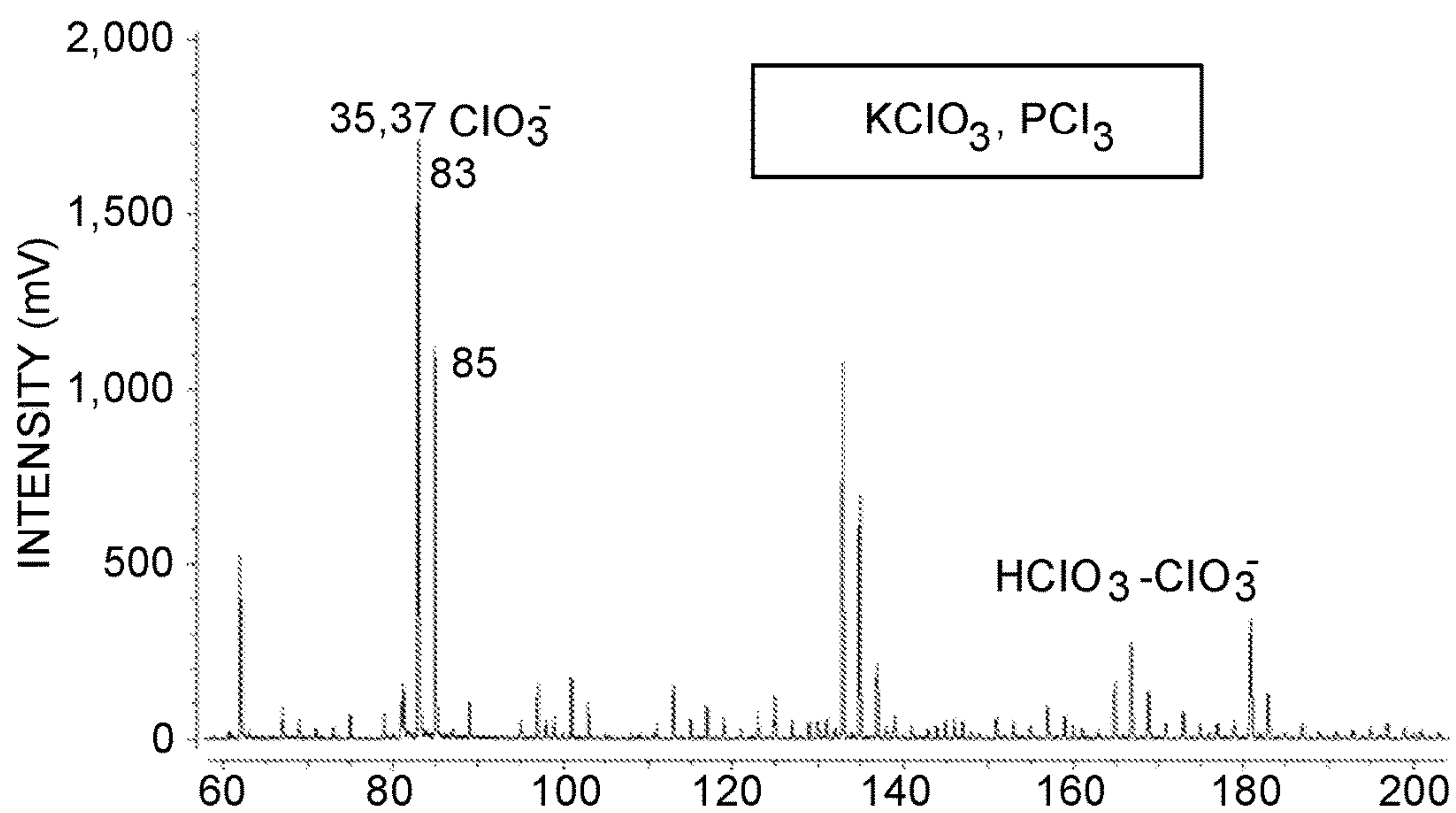
FIG. 11B
